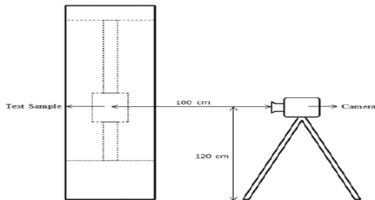
Şekil 3 : Deney düzeneği ve kamera
